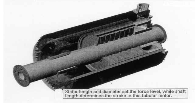
Fig. 2. Linear Motor
